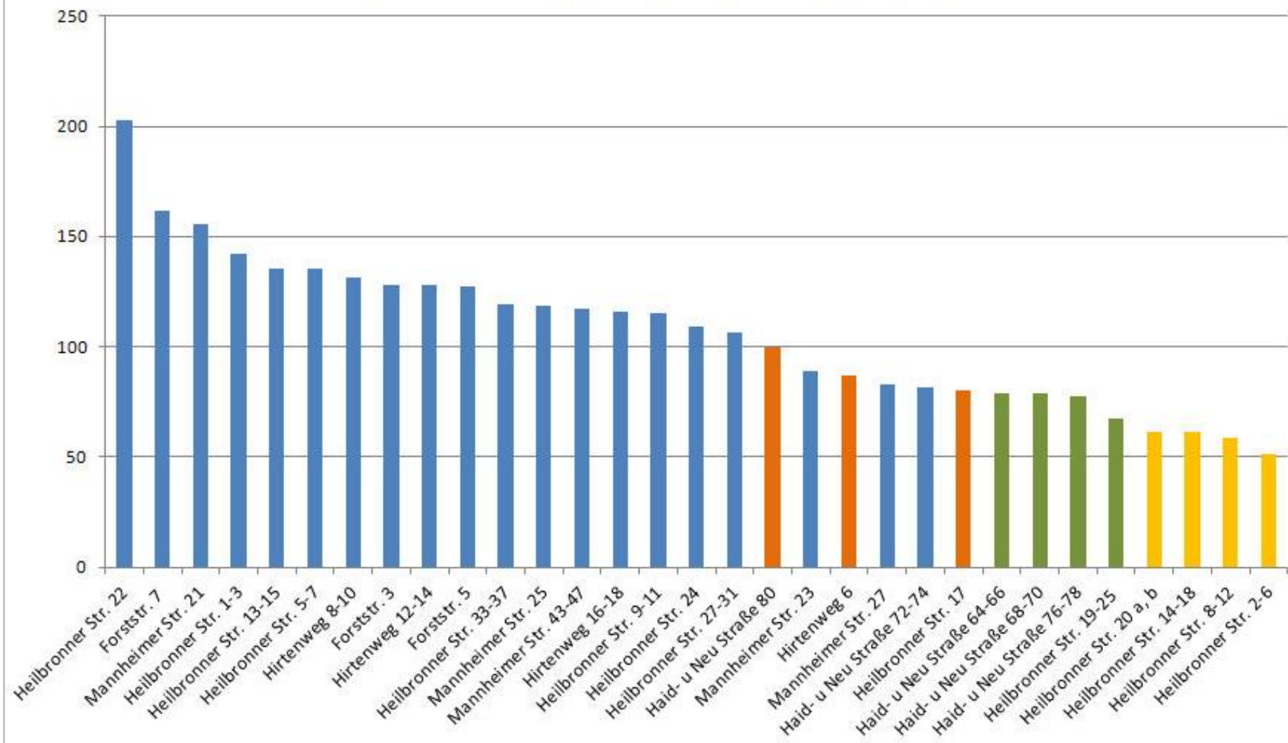
spezif. Wärmeverbrauch (Heizung + WW), Rintheim (kWhth/m 2 )
